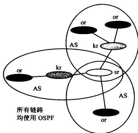
图 2 每个扩散分支属于不同 AS 域
