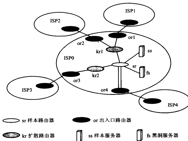
图 1 在一个 ISP 中进行路由扩散网络控管的网络结构
